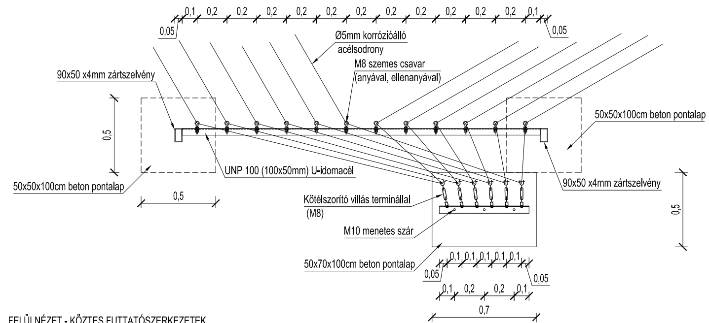
FELÜLNÉZET - KÖZTES FUTTATÓSZERKEZETEK
