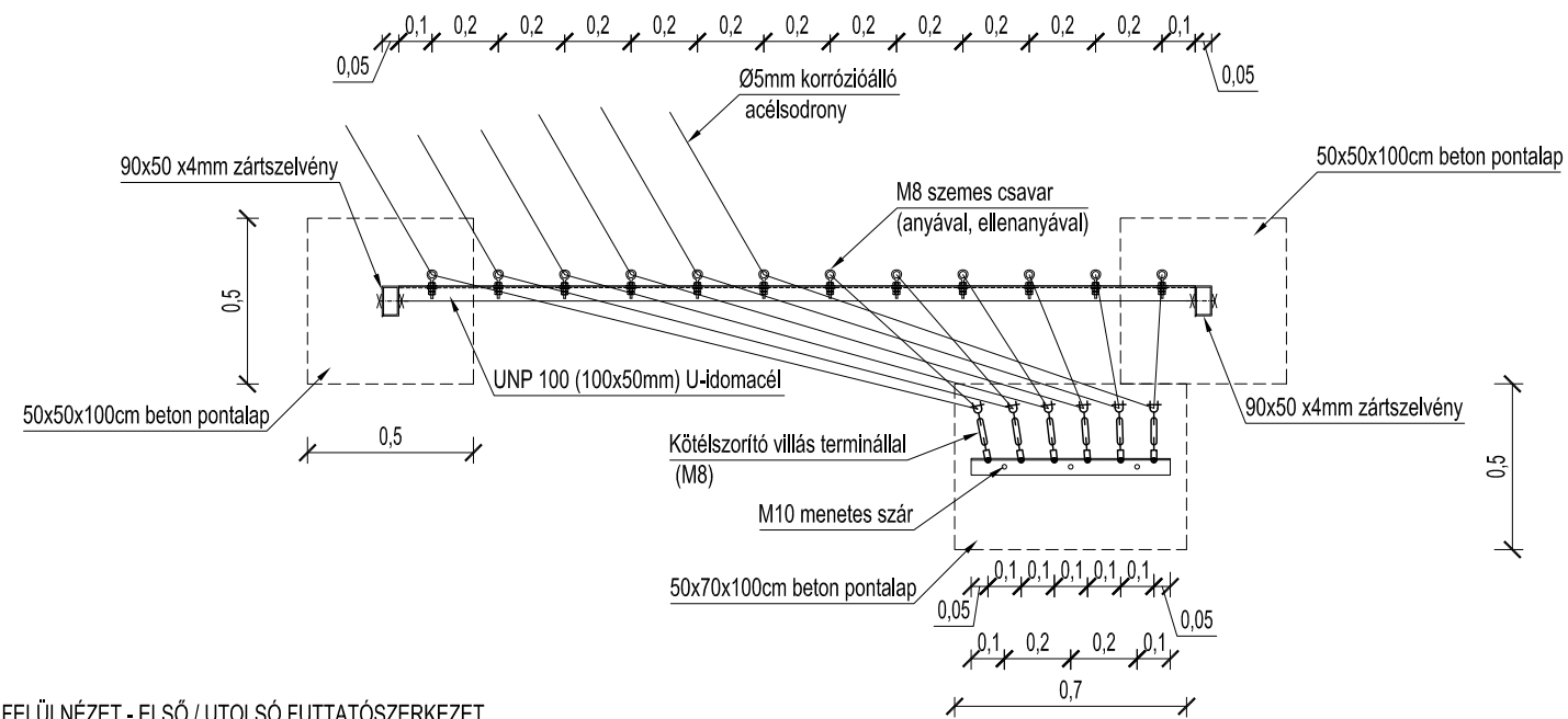
FELÜLNÉZET - ELSŐ / UTOLSÓ FUTTATÓSZERKEZET
