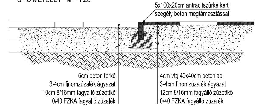
S - S METSZET M = 1:25
