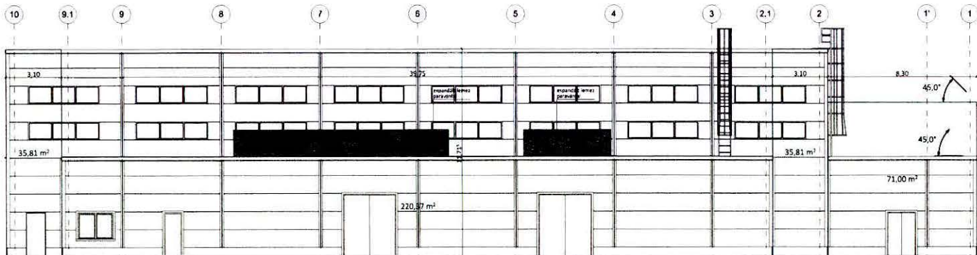
ÉSZAKKELETI HOMLOKZAT m 1:100
