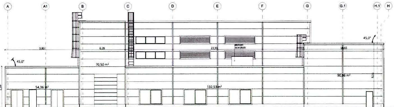
ÉSZAKNYUGATI HOMLOKZAT m 1:100
