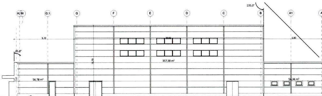
DÉLKELETI HOMLOKZAT m 1:100
