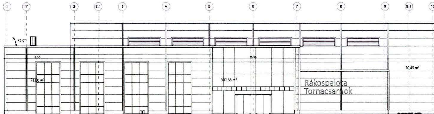
DÉLNYUGATI HOMLOKZAT m 1:100
