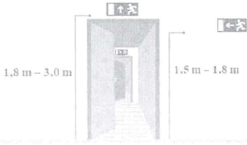
A menekülési jelek elhelyezése
